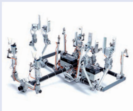
2K-Entnahmegreifer
